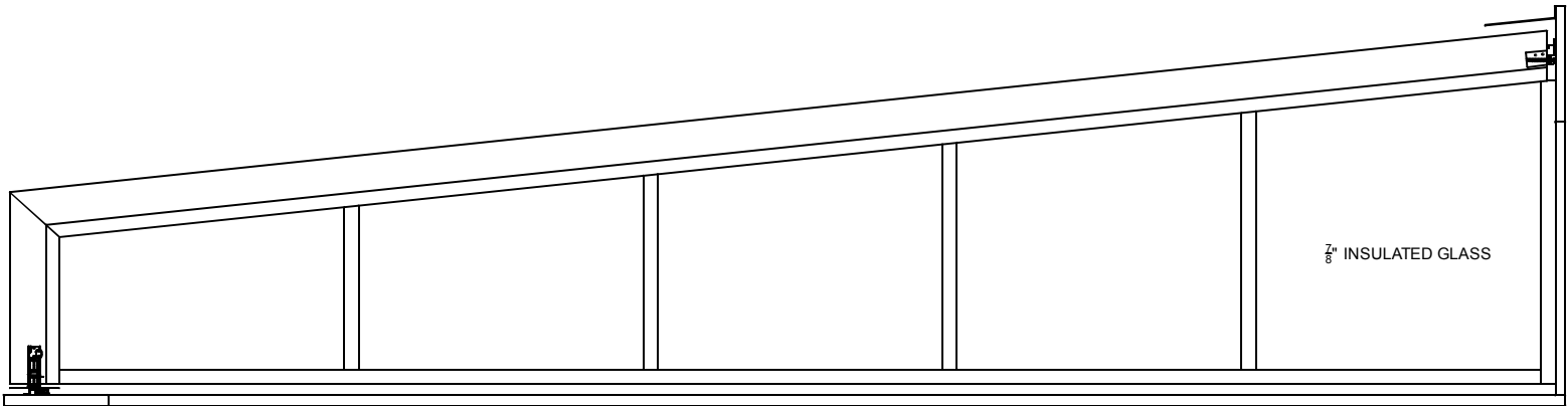
RIGHT ELEVATION
